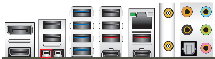
Clear CMOS 按钮
